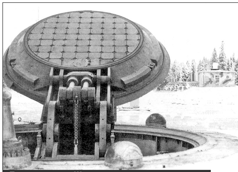
Пуск состоялся. Шахтная пусковая установка для ракеты РС-22А
