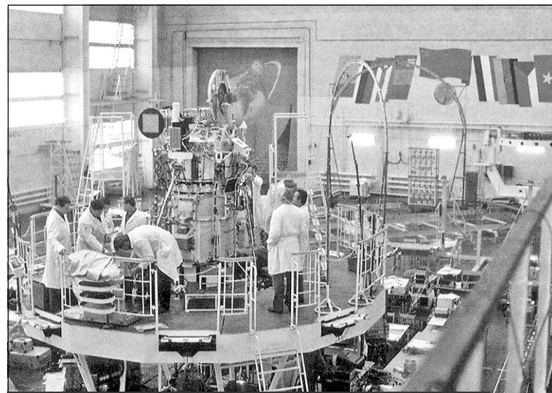
Подготовка КА серии "Интеркосмос" в монтажно-испытательном корпусе космодрома "Плесецк"
