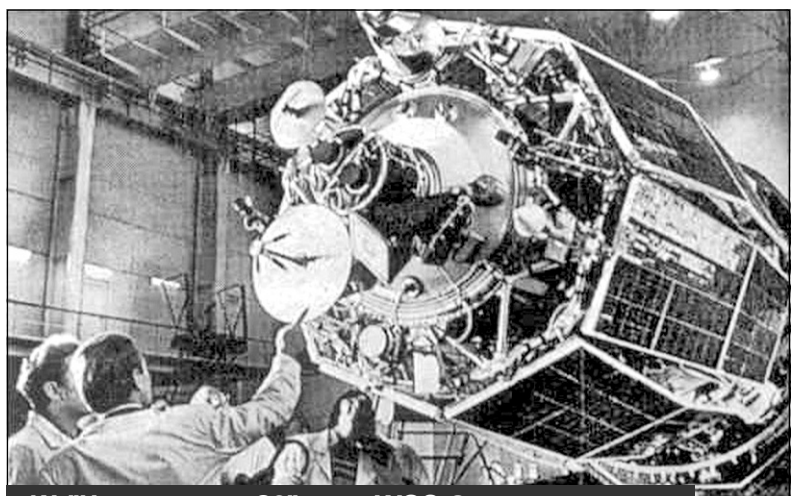
КА "Интеркосмос-20" типа АУОС-3 пристыкован к РН "Космос-3М" в монтажно-испытательном корпусе космодрома "Плесецк"
