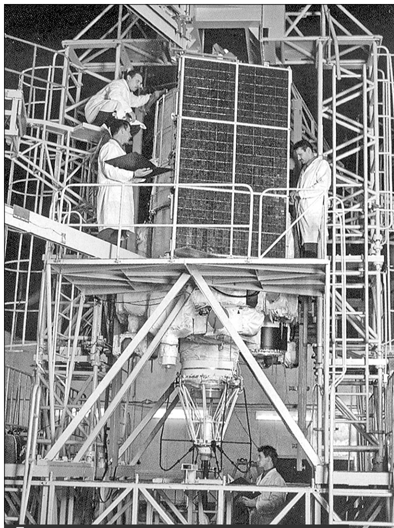
Подготовка к запуску космического аппарата "Метеор-2" в монтажно-испытательном корпусе космодрома "Плесецк"
