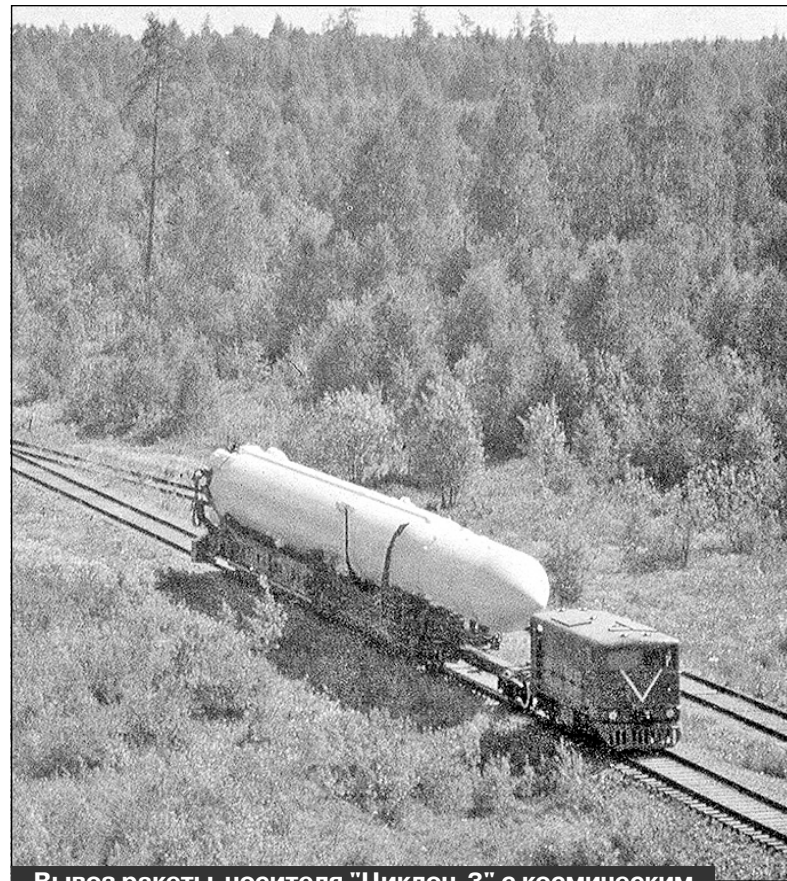
Вывоз ракеты-носителя "Циклон-3" с космическим аппаратом "Муссон" на стартовый комплекс
