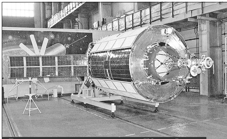
Подготовка космического аппарата "Муссон" к запуску в монтажно-испытательном корпусе
