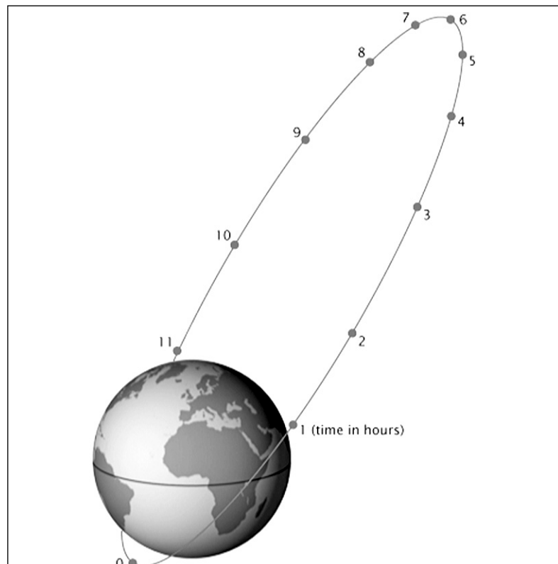
Типичная орбита космического аппарата "Молния-1". Точками отмечено время движения спутника по орбите
