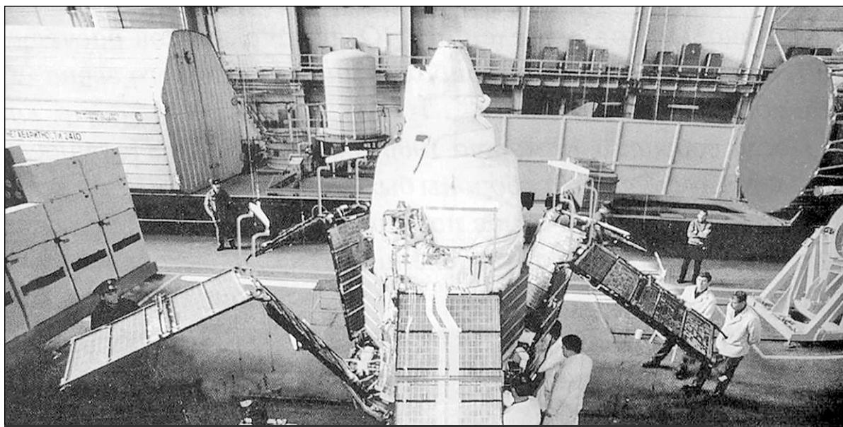
Испытания космического аппарата "Молния-3" на техническом комплексе
