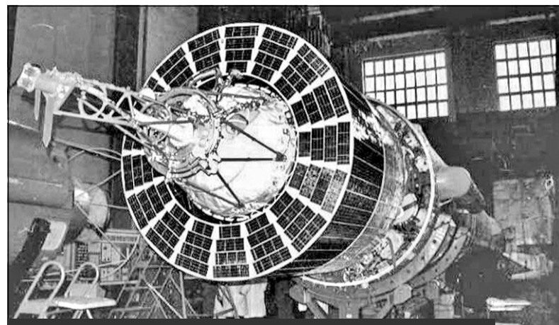
Космический аппарат "Парус"
