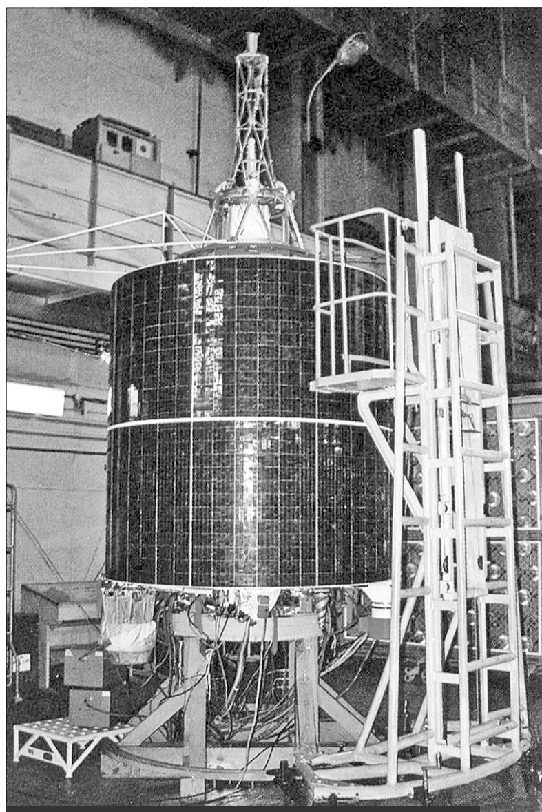
Космический аппарат "Надежда"
