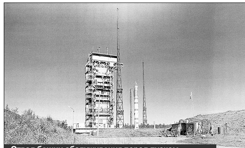
Отвод башни обслуживания перед пуском РН "Космос-3М"
