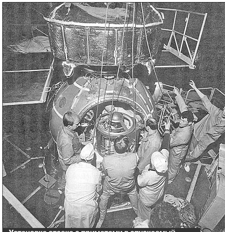
Установка отсека с приматами в спускаемый аппарат КА "Бийон"
