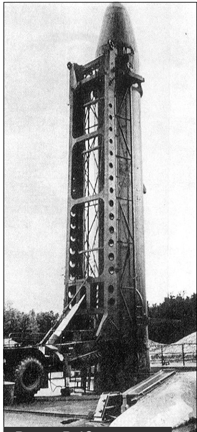
Ракета Р-16 перед установкой в шахту
