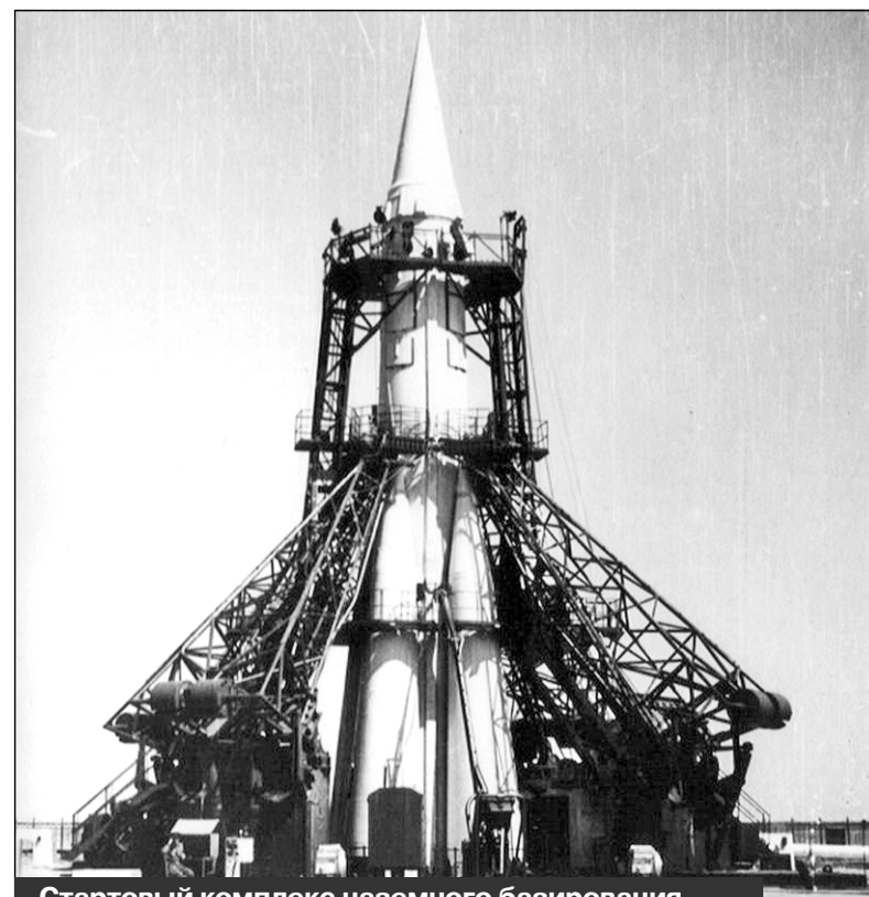
Стартовый комплекс наземного базирования межконтинентальной баллистической ракеты Р-7
