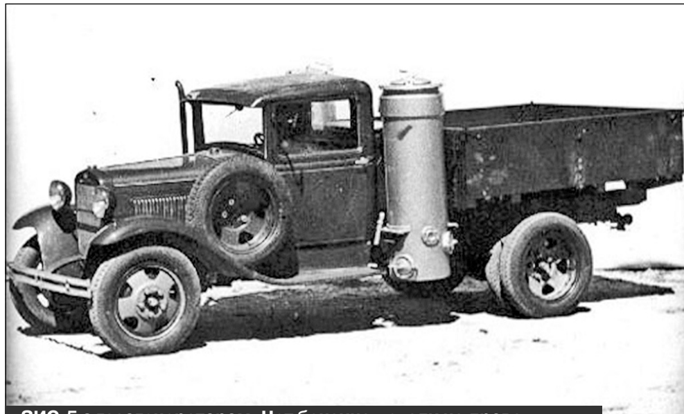
ЗИС-5 с газогенератором. Нет бензина - ехали на дровах. Автомобиль работал на генераторном газе, который получали из древесины
