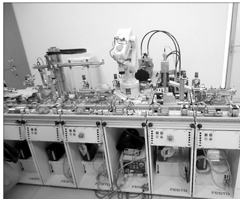
Сборочный станок
