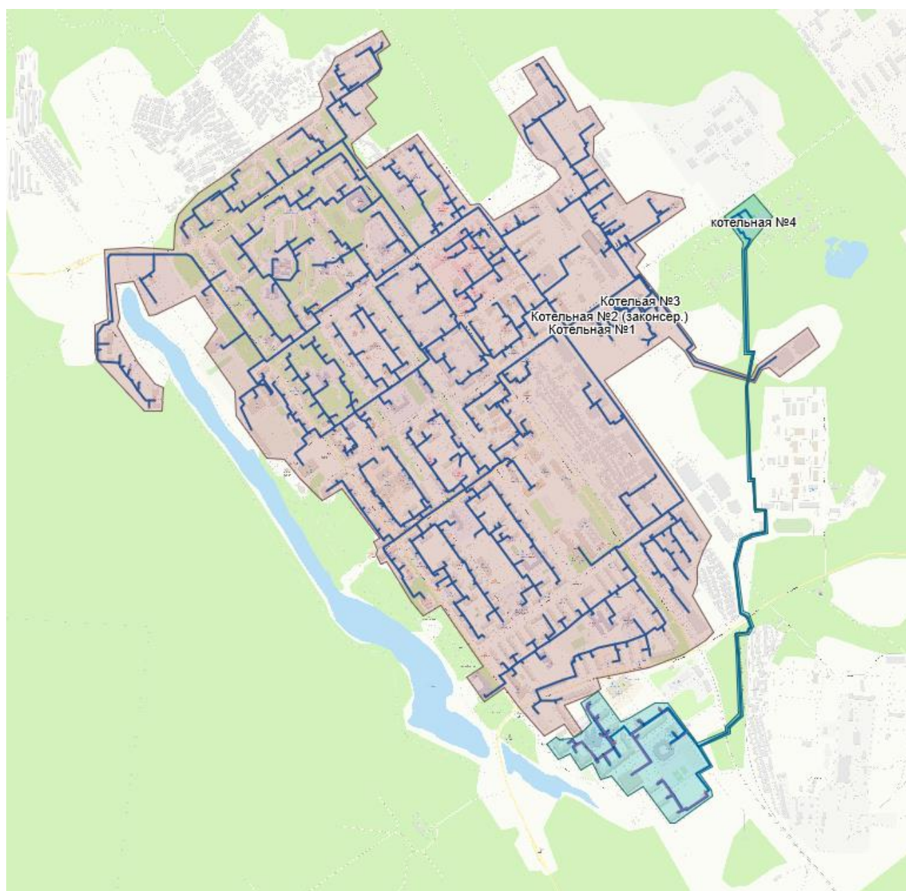
Рисунок 6 – Зона действия источников теплоснабжения г. Мирный
