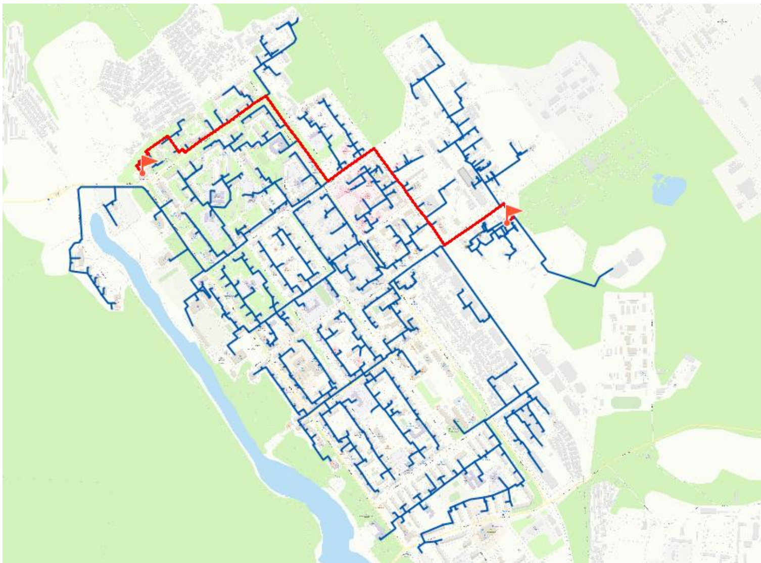
Рисунок 8 – Путь для расчёта вероятности безотказной работы тепловых (расчетный путь №4)
