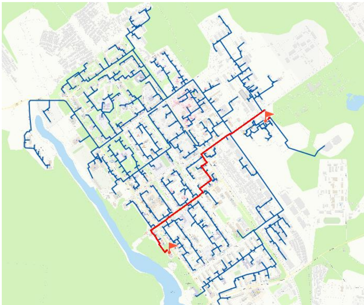
Рисунок 10 – Путь для расчёта вероятности безотказной работы тепловых (расчетный путь №4)
