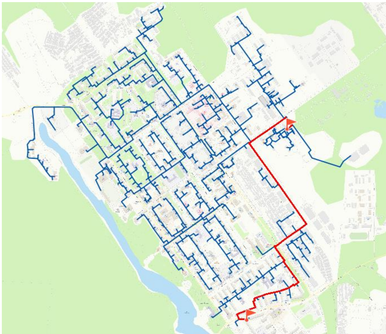
Рисунок 11 – Путь для расчёта вероятности безотказной работы тепловых (расчетный путь №5)
