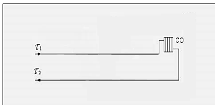
Рисунок 2 - Схема подключения потребителей к двухтрубной тепловой сети (при наличии внутренней системы отопления), зависимое присоединение, без смешения
