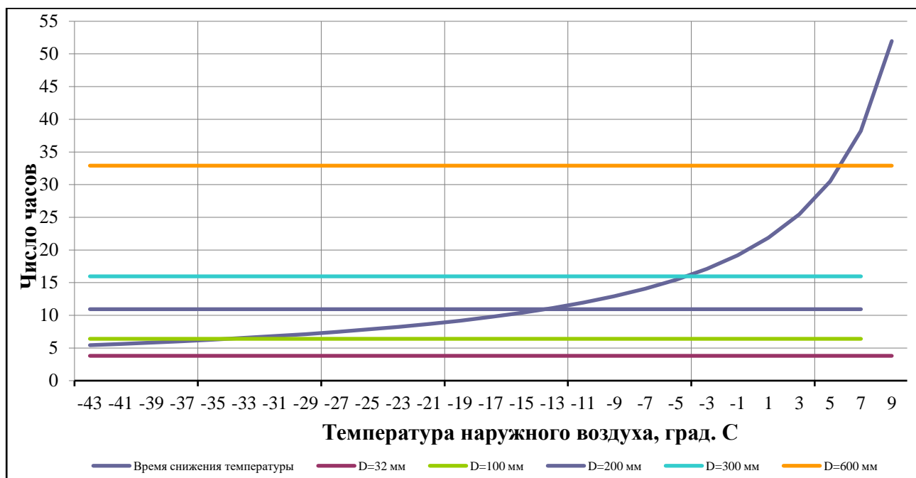
Рисунок 13 - Графическое сравнение периода времени снижения температуры внутреннего воздуха до критического значения и периода времени, необходимого для восстановления участка тепловой сети
