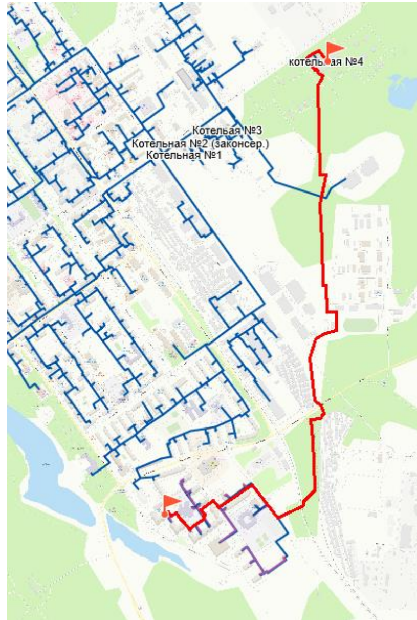
Рисунок 12 – Путь для расчёта вероятности безотказной работы тепловых (расчетный путь №5)
