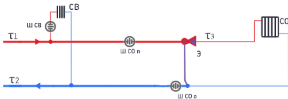
Рисунок 3 – Схема подключения потребителей к двухтрубной тепловой сети (при наличии внутренней системы отопления), в качестве регулятора температуры используется элеватор (СО – система отопления, Э – элеватор, СВ – система вентиляции)
