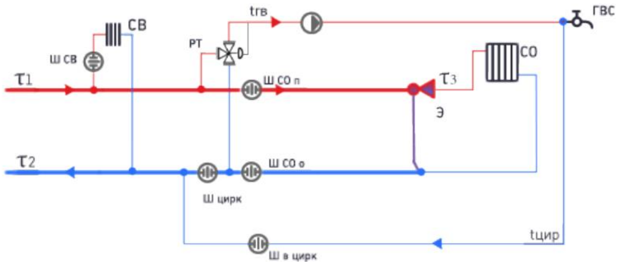
Рисунок 5 – Потребитель с открытым водоразбором на ГВС и элеваторным присоединением СО
