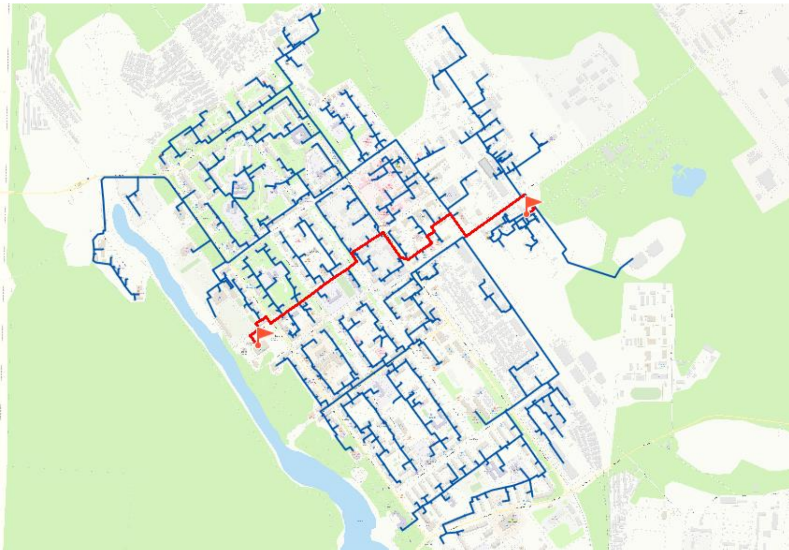
Рисунок 9 – Путь для расчёта вероятности безотказной работы тепловых (расчетный путь №3)
